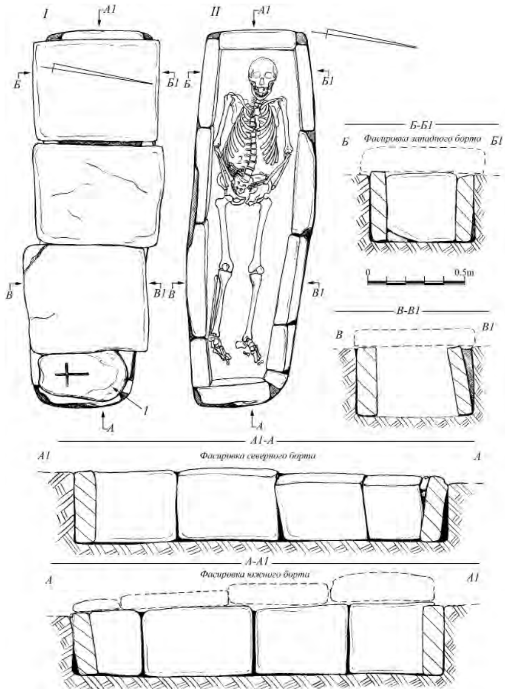
Рис. 4. Могила 37. Планы плитового перекрытия (I) и погребения (II), разрезы к планам и фасировки бортов.
