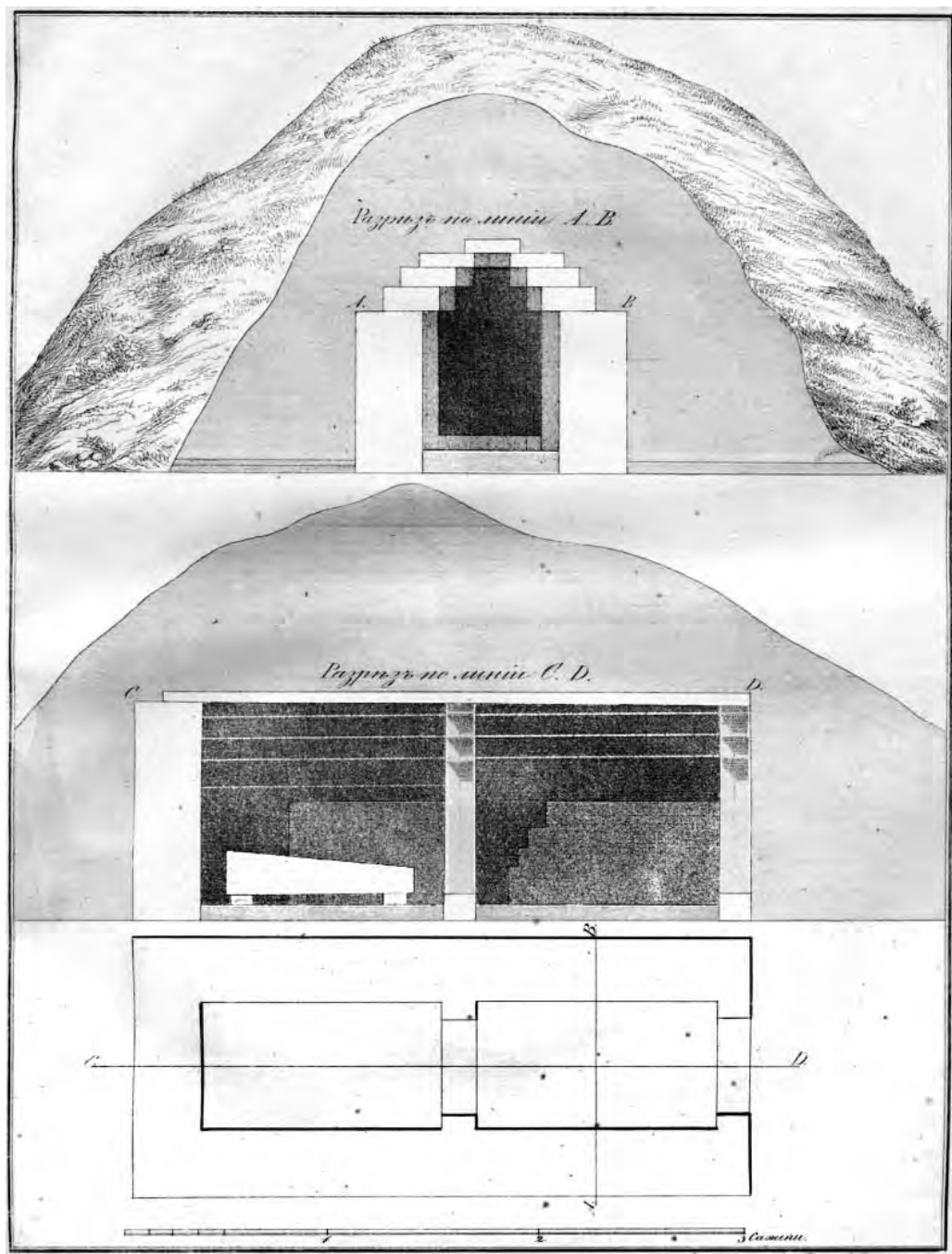
Рис. 21. Склеп 1841 г., открытый А.Б. Ашиком в кургане около дороги на Аджимушкайские каменоломни (по Ашик, 1848).
