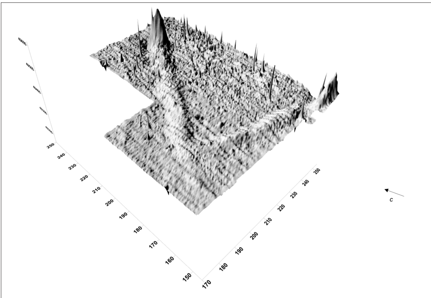
Рис. 9. Юго-западная часть оборонительных сооружений Лабриса (Семибратного городища). Трехмерная модель магнитных аномалий.
