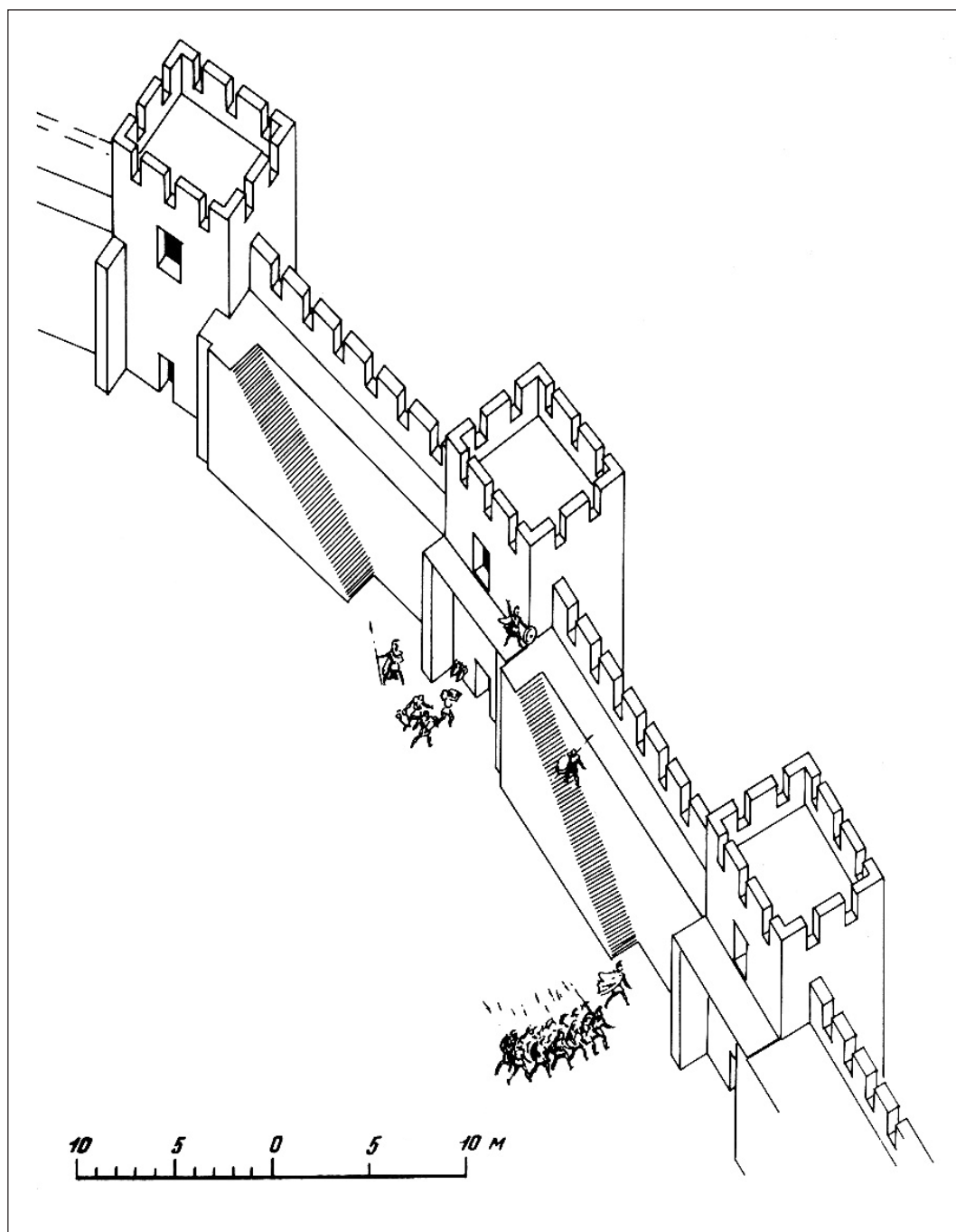
Рис. 4. Реконструкция северо-восточной оборонительной линии Семибратнего городища (по В.П. Толстикову).
