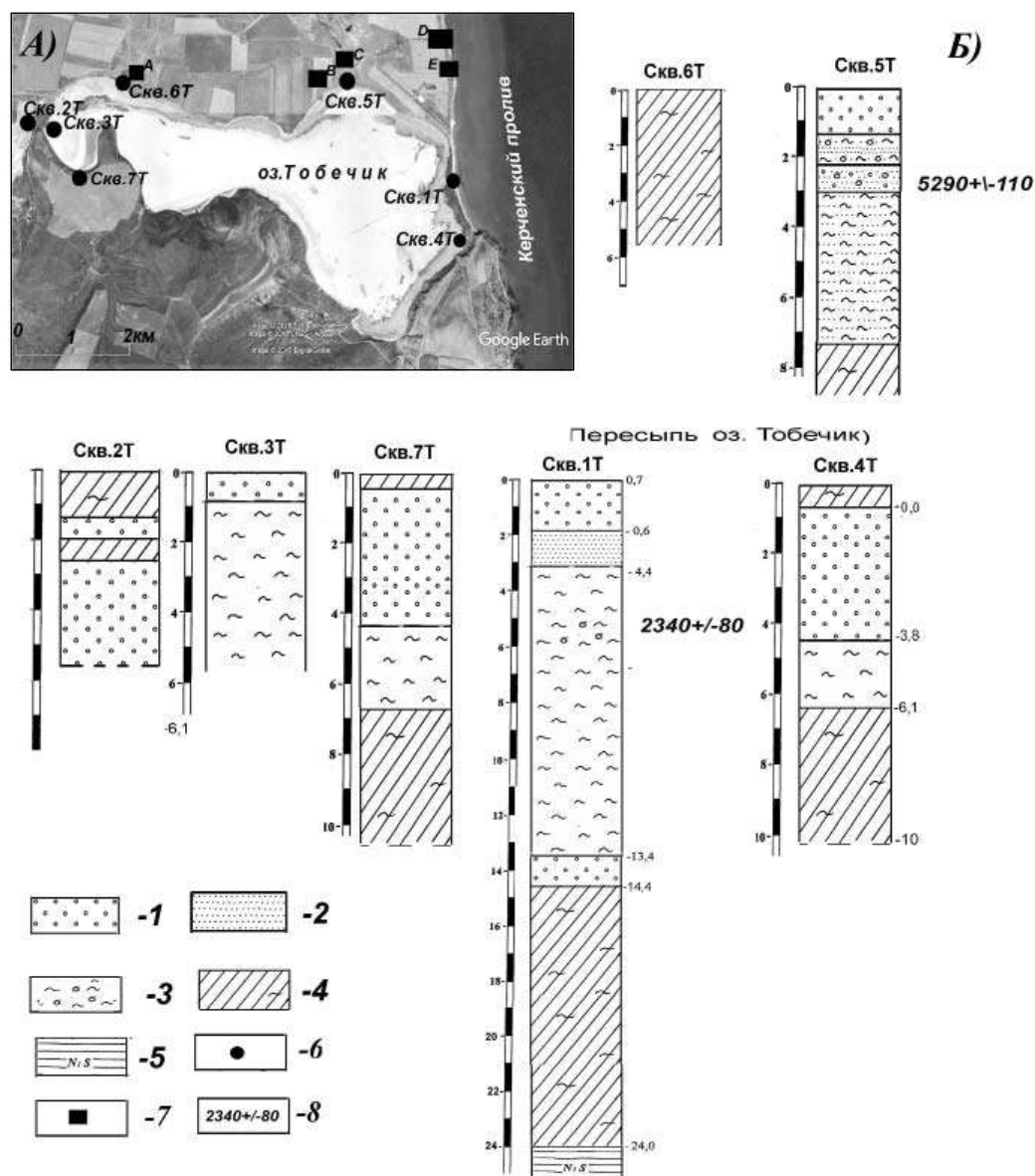
Рис. 1. Расположение скважин и поселений античного времени (А) и строение прибрежных отложений на побережье оз. Тобечик (Б).
