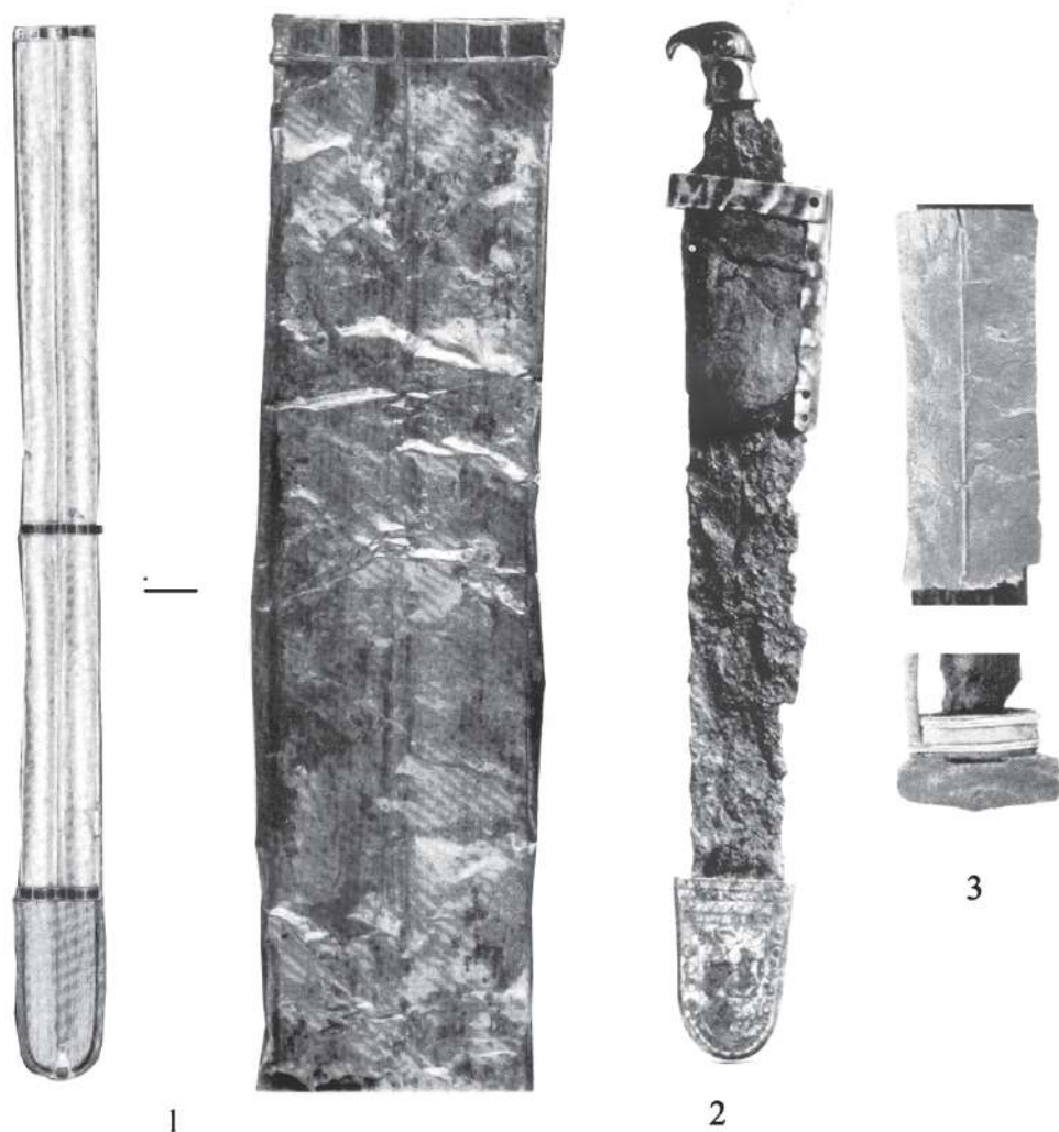
Рис. 7. Короткие мечи и боевые ножи Боспора Киммерийского и детали меча из Альтлюсхейма.
