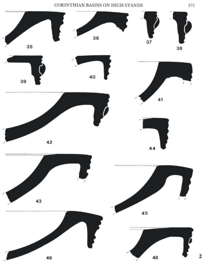
FIG. 2. Profiles. Scale 1:2
