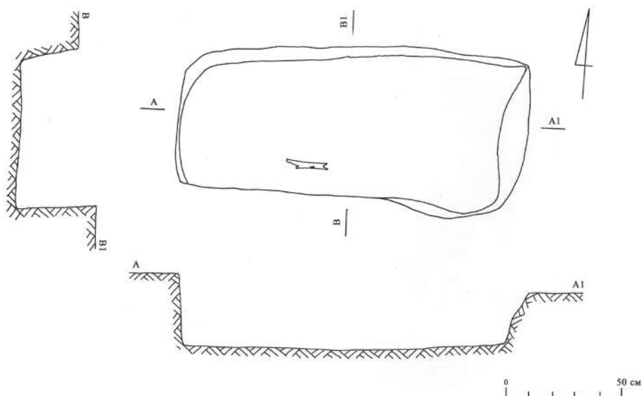
Рис.23. План и разрезы могилы М-010/2022.
