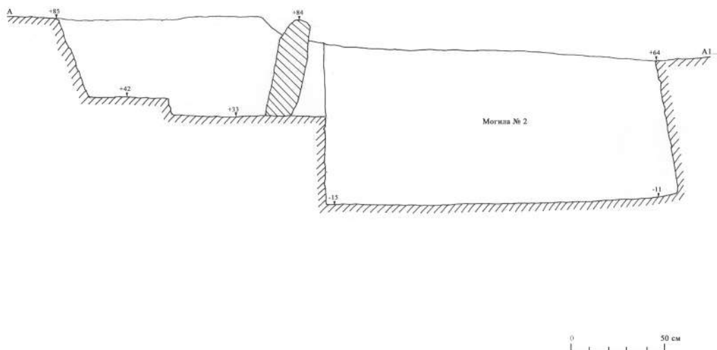
Рис.8. Разрез А-А1 могилы М-02/2022 (склеп).
