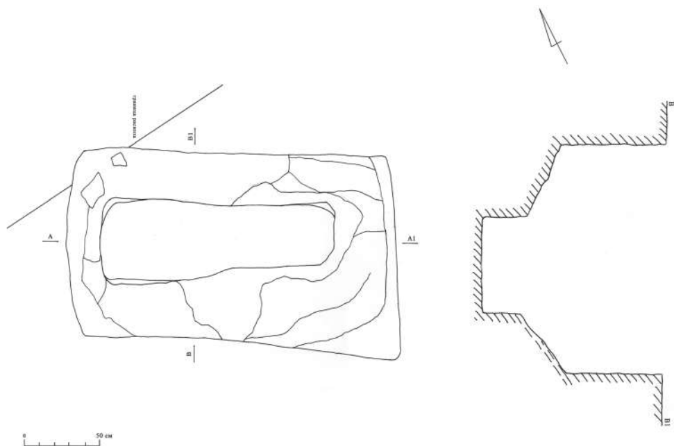
Рис.19. План и разрез могилы М-07/2022.
