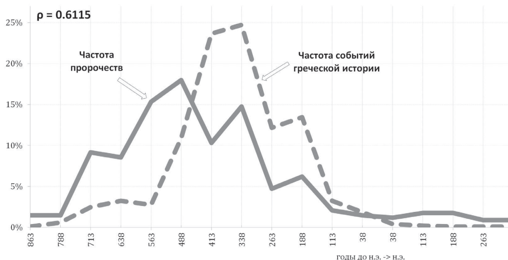
Рис. 2. Колебания частоты дельфийских пророчеств по 75-летним отрезкам на фоне основных событий греческой истории IX в. до н.э. - IV в. н.э. (по: Parke, Wormell, 1956; Fontenrose, 1978, Бикерман, 1975, табл. XI).
